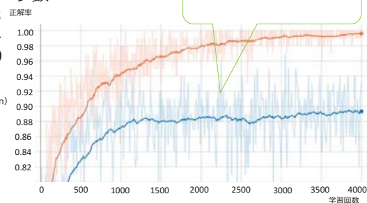
図7 分割前の画像の学習結果
